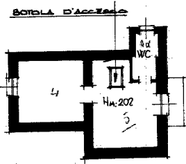
PIANO SECONDO
