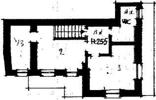
PIANO PRIMO
